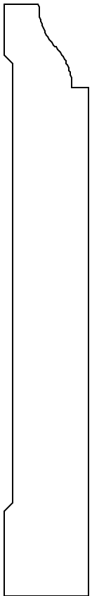
OB1063 5/8 X 4-3/8
