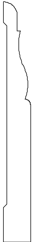
OB1069 1/2 X 4-3/8
