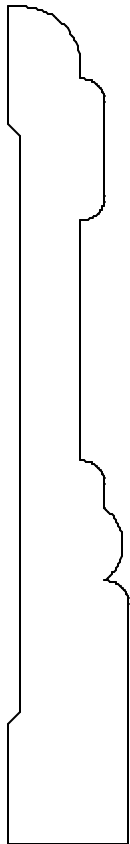
OB1038 5/8 X 4-3/8
