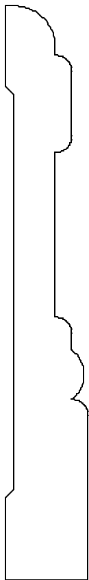
OB1038 5/8 X 4-3/8
